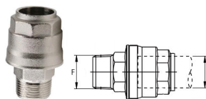
RACCORDO DRITTO MASCHIO - NPTF
