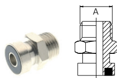
RACCORDO MASCHIO A BAIONETTA
