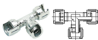
RACCORDO T CON DADI CAPETTATI
