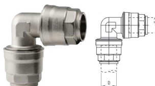
RACCORDO A "L" INTERMEDIO
