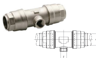
RACCORDO PER CALATA FEMMINA
