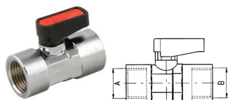
VALVOLA FEMMINA RP ISO 7 - FEMMINA RP ISO 7
