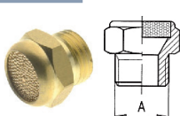
SILENZIATORE A RETE IN OTTONE 100 MICRON
