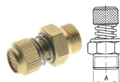
SILENZIATORE REGOLABILE 100 MICRON OTTONE
