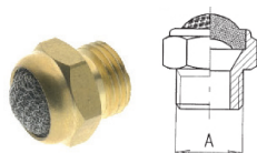
SILENZIATORE IN OTTONE CON RETE IN FILO DI ACCIAIO INOX 304
