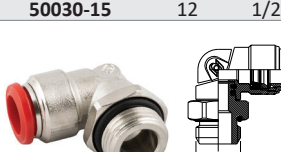
RACCORDO A L ORIENTABILE MASCHIO CILINDRICO - METRICO
