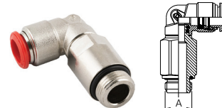
RACCORDO A L ORIENTABILE PROLUNGATO MASCHIO CILINDRICO
