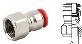
RACCORDO DIRITTO FEMMINA CILINDRICO
