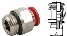
RACCORDO DIRITTO MASCHIO CILINDRICO - METRICO
