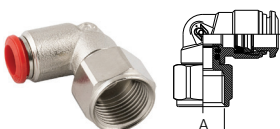
RACCORDO A L ORIENTABILE FEMMINA
