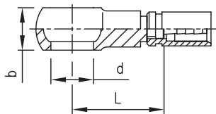
RACCORDO A OCCHIO DRITTO - DIN 7642
