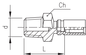
RACCORDO MASCHIO FISSO CONICO NPT
