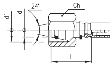
RACCORDO FEMMINA METRICA GIREVOLE 24° CON O-RING - ISO 12151-2
