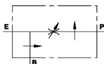
VALVOLA PRIORITARIA A 3 VIE CON TERZA VIA IN PRESSIONE - VPR3
