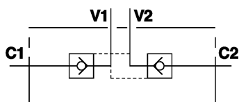
VALVOLE DI BLOCCO PILOTATE A DOPPIO EFFETTO CON 2 CART. EXTRA CORTE - VBPDE 2 CEXC
