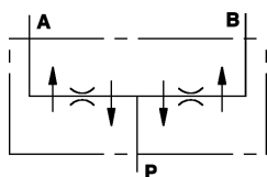
VALVOLE EQUILIBRATRICI DI FLUSSO A 2 VIE IN ACCIAIO - DFL
