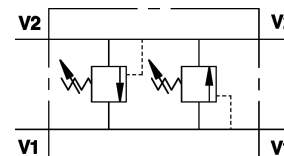
VALVOLA ANTIURTO - VAU
