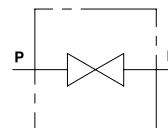
ESCLUSORE MANOMETRO IN LINEA E 90° - EML
