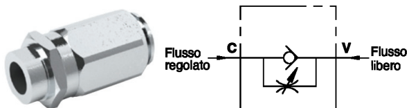
VALVOLE DI REGOLAZIONE FLUSSO UNIDIREZIONALI A MANICOTTO - VRF
