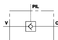
VALVOLE DI BLOCCO PILOTATE A SEMPLICE EFFETTO A 3 VIE IN LINEA - VBPDE 2 CEXC
