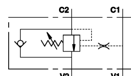
VALVOLA DI BLOCCO E CONTROLLO DISCESA SEMPLICE EFFETTO TIPO A - VBCD SE A
