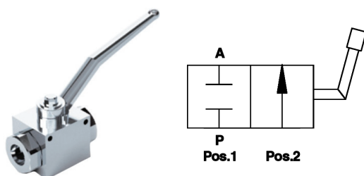
RUBINETTO A SFERA A 2 VIE - RS 2
