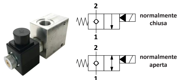
VALVOLA A CARTUCCIA - SVCP
