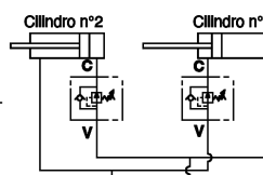
VALVOLE DI SEQUENZA AD AZIONE DIRETTA - V2SC
