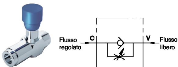
VALVOLE DI REGOLAZIONE FLUSSO UNIDIREZIONALI A 90° - VRFU
