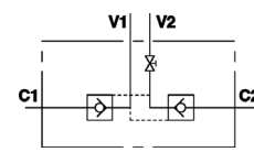
VALVOLE DI BLOCCO PILOTATE A DOPPIO EFFETTO CON RUBINETTO - VBPDE c/RUB.
