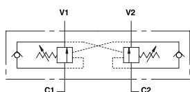
VALVOLA DI BLOCCO E CONTROLLO DISCESA A DOPPIO EFFETTO A FLANGIA - VBCD DE FL
