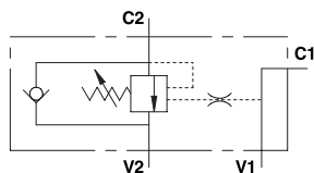
VALVOLA DI BLOCCO E CONTROLLO DISCESA A SEMPLICE EFFETTO A FLANGIA - VBCD SE FL
