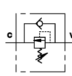
VALVOLE DI SEQUENZA AD AZIONE DIRETTA - V2SC
