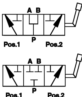
DEVIATORI DI FLUSSO A 3 VIE ALTA PRESSIONE IN ACCIAIO - DF 3 AP
