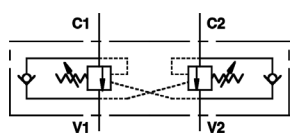
VALVOLA DI BLOCCO E CONTROLLO DISCESA DOPPIO EFFETTO - VBCD DE
