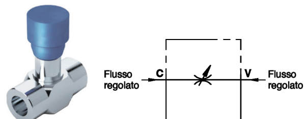
VALVOLE DI REGOLAZIONE FLUSSO BIDIREZIONALI A 90° - VRFB
