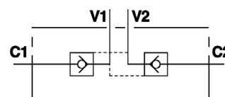
VALVOLE DI BLOCCO PILOTATE A DOPPIO EFFETTO COMPATTE - CMP/FLV - VBPDE
