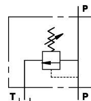
VALVOLE DI MASSIMA PRESSIONE AD AZIONE DIRETTA IN LINEA - PESANTE - VMP
