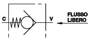
VALVOLE UNIDIREZIONALI - VU
