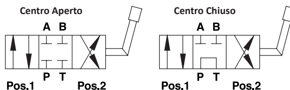
DEVIATORI DI FLUSSO A 4 VIE - CORPO IN GHISA - IF 4
