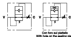
VALVOLE UNIDIREZIONALI CON BLOCCO AUTOMATICO "PARACADUTE" - FLIP/FLOP - VUBA
