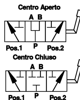
DEVIATORI DI FLUSSO A 3 VIE - CORPO IN GHISA - DF 3
