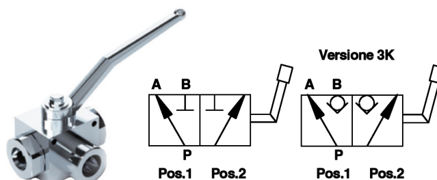
RUBINETTO A SFERA A 3 VIE - RS 3
