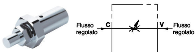
VITE STROZZATRICE - VS
