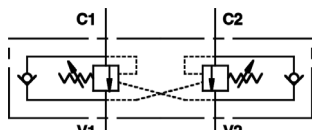
VALVOLA DI BLOCCO E CONTROLLO DISCESA DOPPIO EFFETTO TIPO A - VBCD DE A
