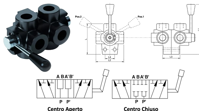
DEVIATORI DI FLUSSO A 6 VIE - DF 6
