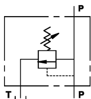
VALVOLE DI MASSIMA PRESSIONE AD AZIONE DIRETTA IN LINEA - LEGGERA - VMP L
