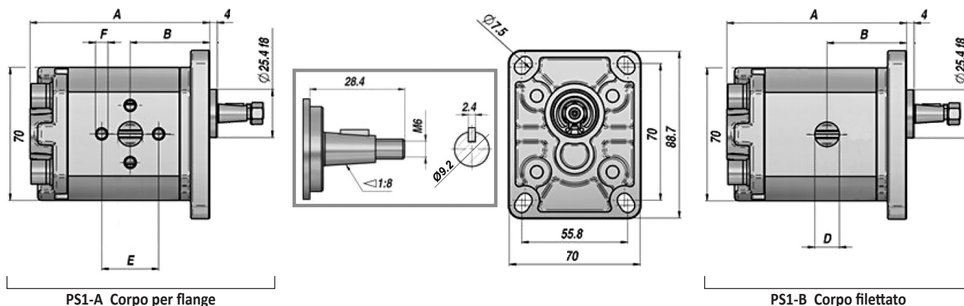
PS1-A Corpo per flange
