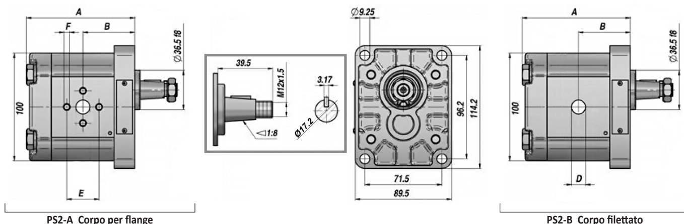
PS2-A Corpo per flange
