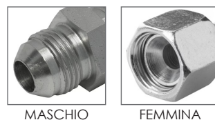
JIC 37°
