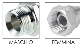
METRIC 60°
