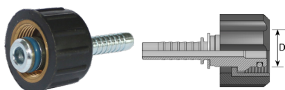
FEMMINA PER IDROPULITRICI TIPO "FK"
